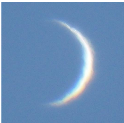
Foto 1: Venere prima della congiunzione eliaca.
